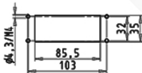
Bohrbild /Cut out
