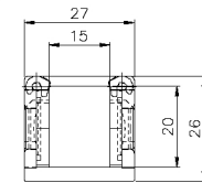
SECTION A-A (S=2:1)
